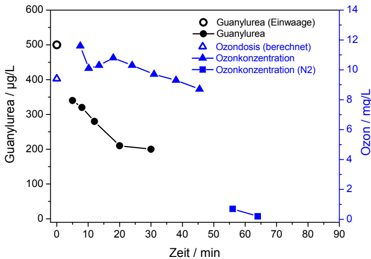
Abb. 41: Abnahme von Guanylarnstoff während der Ozonung
