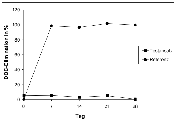
Abb. 23: DOC-Elimination von Formylaminoantipyridin im Zahn-Wellens-Test
